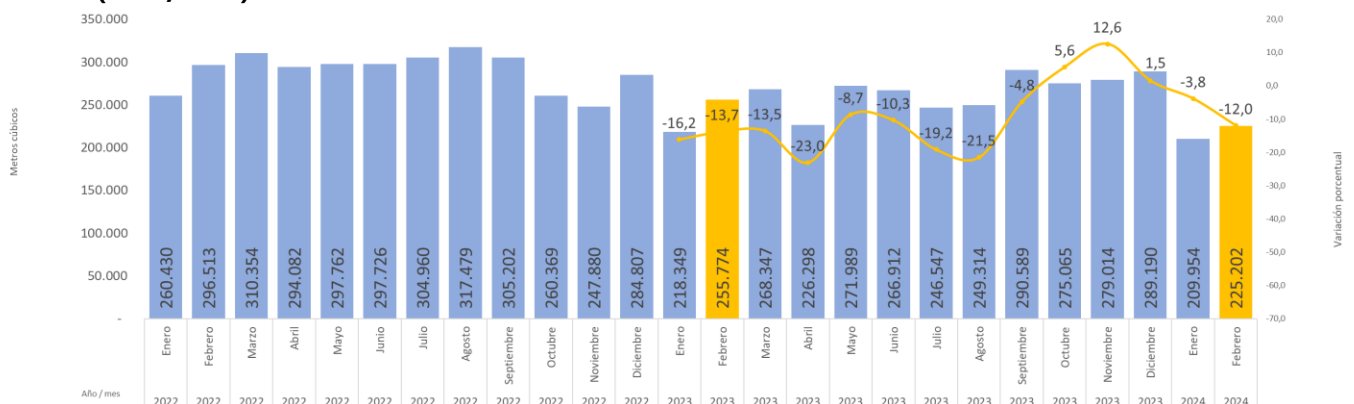
Gráfica 1. Producción de mezcla asfáltica (metros cúbicos y variación anual)
