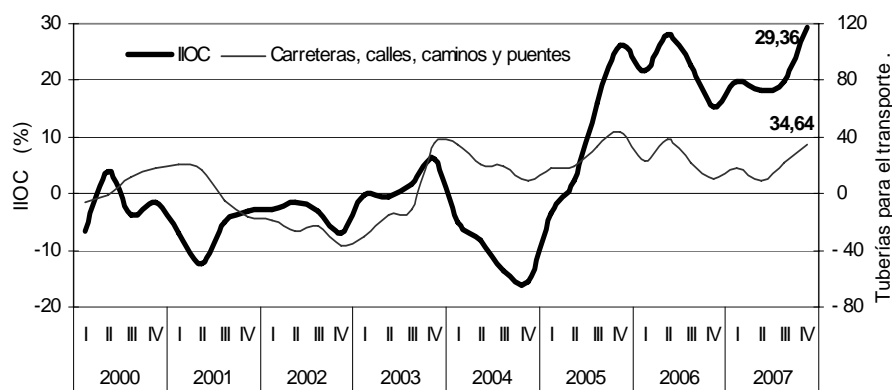
Gráfico 3.4 IIOC total e IIOC carreteras, calles, caminos y puentes Variación doce meses 2000 (I trimestre) - 2007 (IV trimestre) p
