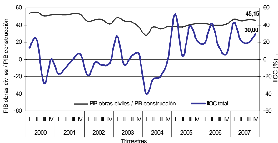
Gráfico 3.1 Participación del PIB de obras civiles en el PIB de construcción y variación anual del IIOC 2000 (I trimestre) - 2007 (IV trimestre) P
