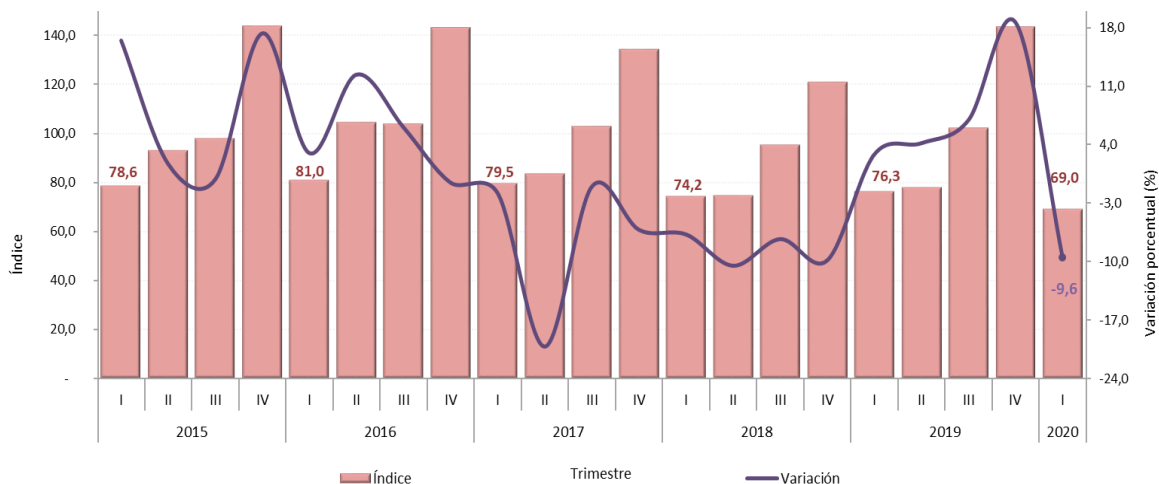
Gráfico 5. Índice y variación anual de los pagos de vías de agua, puertos, represas, acueductos, alcantarillado y otras obras portuarias Total nacional – serie empalmada 2015 – 2020 Pr (I trimestre)
