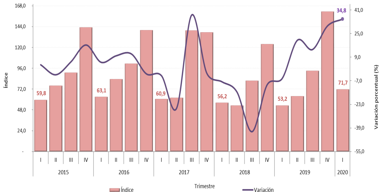
Gráfico 10. Índice y variación anual de las obligaciones de vías de agua, puertos, represas, acueductos, alcantarillados y otras obras portuarias Total nacional – serie empalmada 2015 – 2020 Pr (I trimestre)
