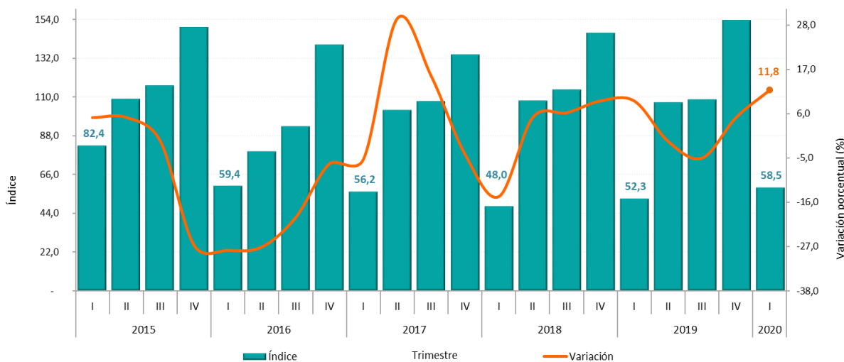
Gráfico 9. Índice y variación anual de las obligaciones de construcciones para la minería, centrales generadoras eléctricas y tuberías para el transporte a larga y corta distancia Total nacional – serie empalmada 2015 – 2020 Pr (I trimestre)
