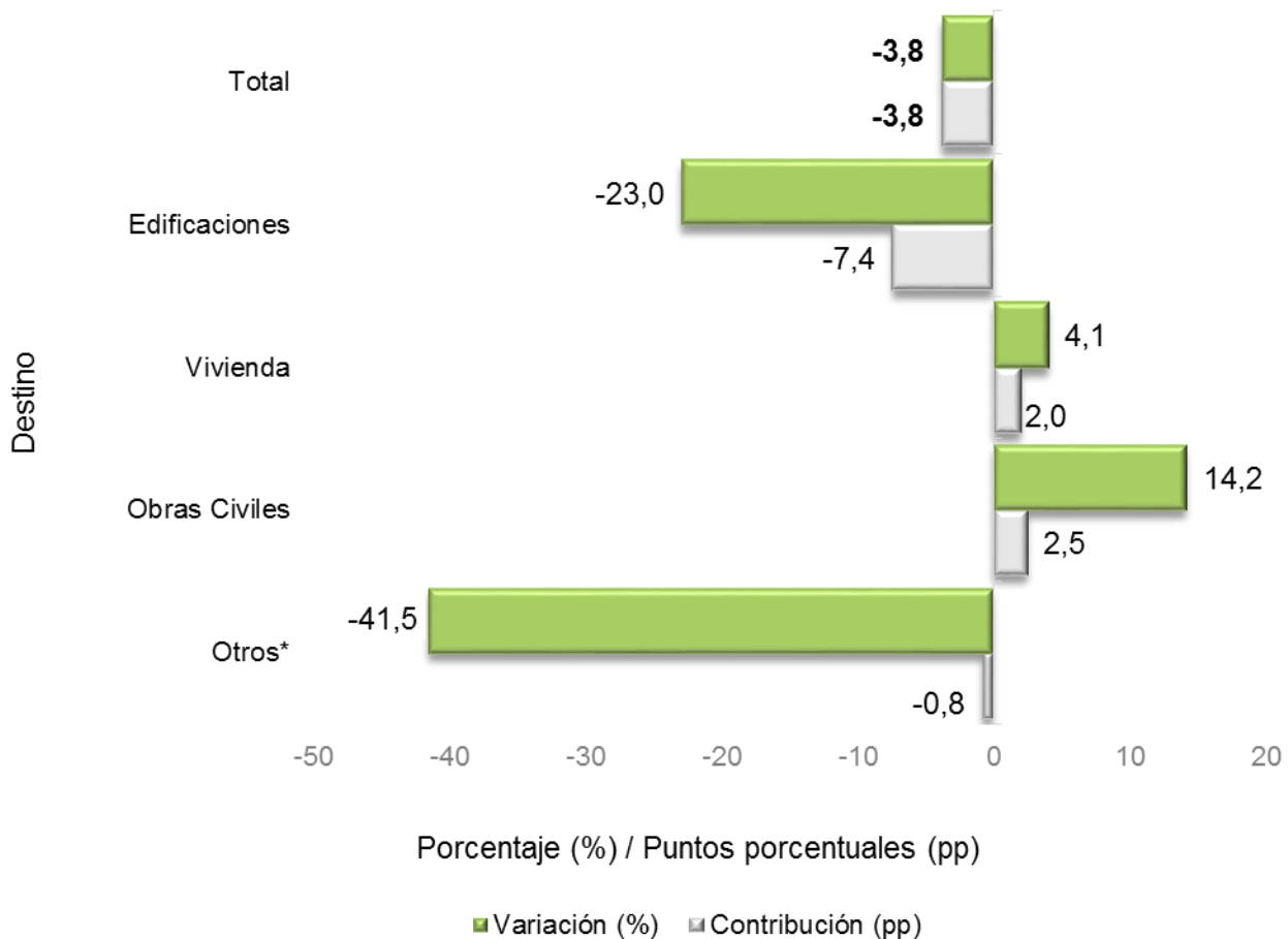
Gráfico 8. Variación y contribución anual del concreto premezclado, según destino Total nacional Noviembre (2017 P / 2016)
