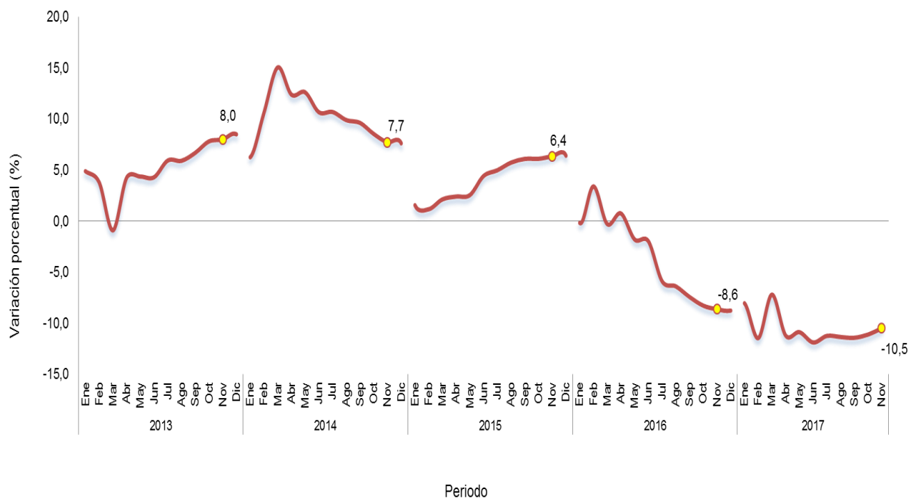
Gráfico 4. Variación año corrido del concreto premezclado Total nacional 2013 (enero) – 2017 (noviembre) P
