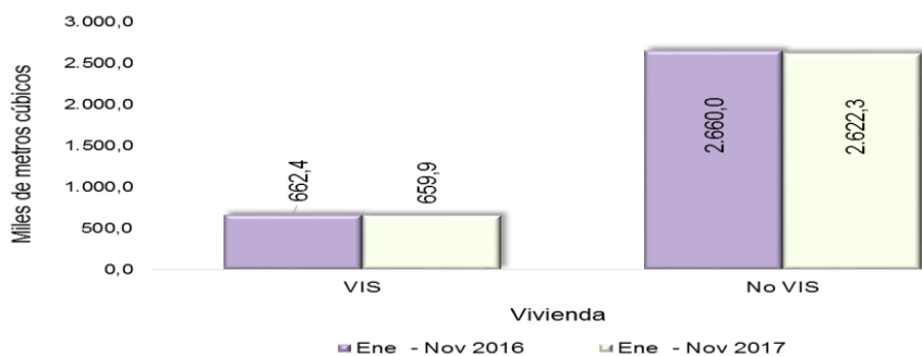
Gráfico 15. Concreto premezclado destinado a vivienda (VIS y No VIS) Total nacional Enero – noviembre (2017 p / 2016)
