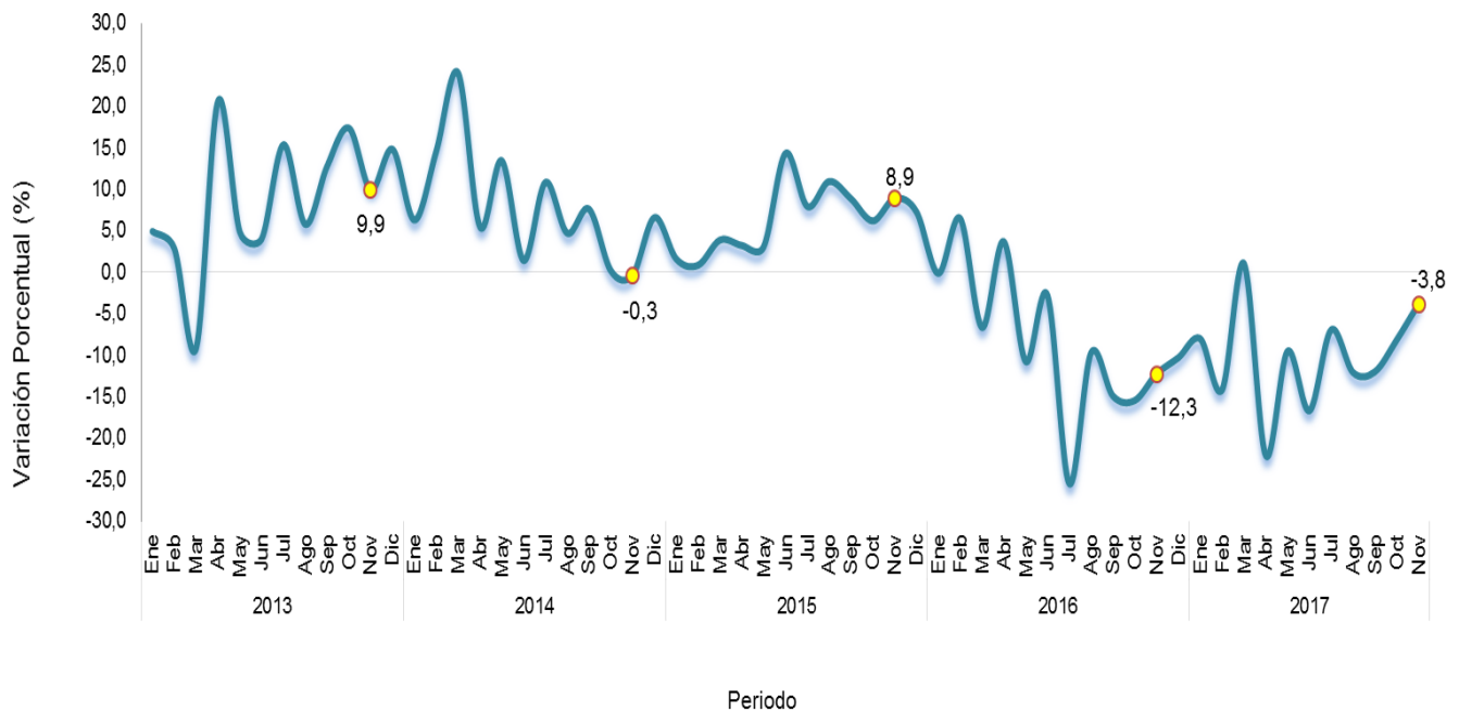
Gráfico 2. Variación anual del concreto premezclado Total nacional 2013 (enero) – 2017 (noviembre) P
