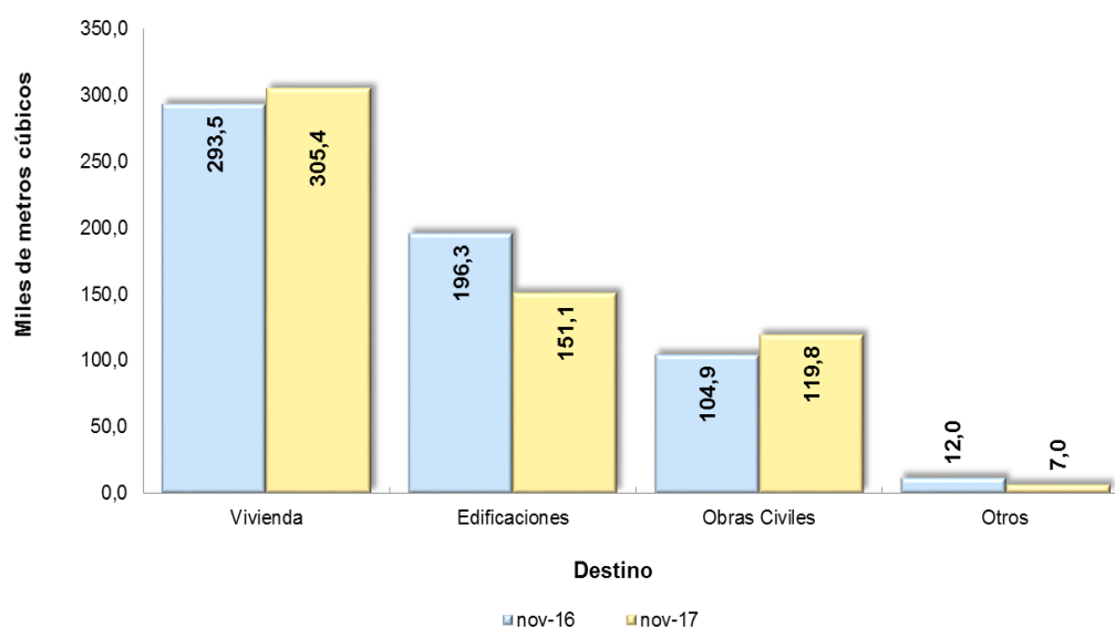
Producción anual de concreto premezclado según destinos Total nacional Noviembre (2016 - 2017)
