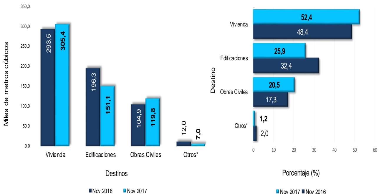
Gráfico 7. Producción y distribución porcentual de concreto premezclado según destino Total nacional Noviembre (2017 P / 2016)
