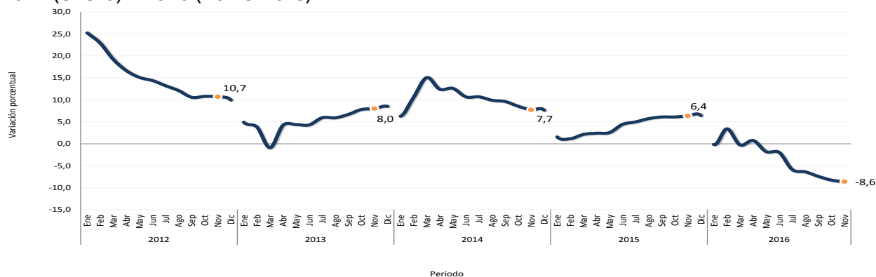
Gráfico 4. Variación año corrido del concreto premezclado Total nacional 2012 (enero) – 2016 (noviembre) P
