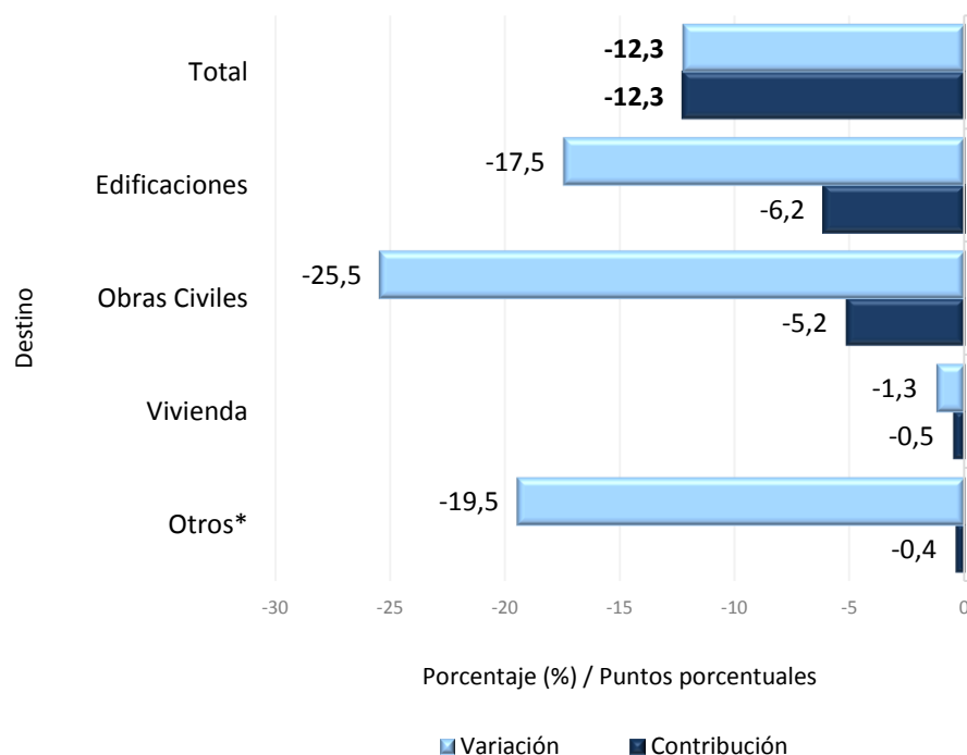
Gráfico 8. Variación y contribución anual del concreto premezclado, según destino Total nacional Noviembre 2016 P / 2015
