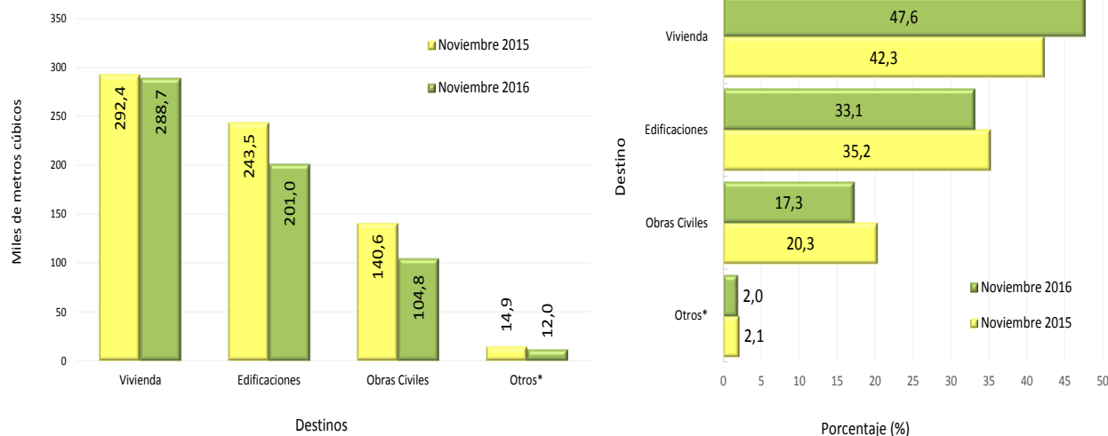
Gráfico 7. Producción y participación anual de concreto premezclado según destino Total nacional Noviembre 2016 P / 2015
