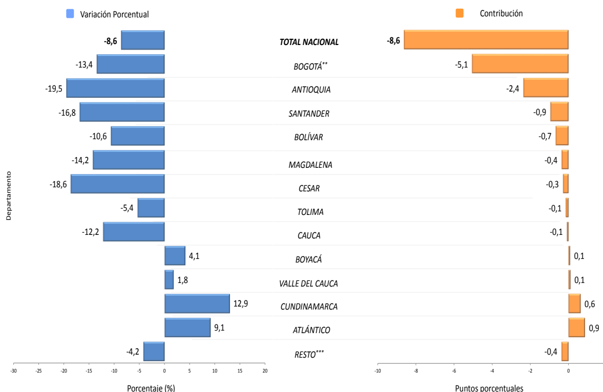
Gráfico 20. Variación año corrido del concreto premezclado, según departamentos Enero - noviembre 2016 P / enero - noviembre 2015
