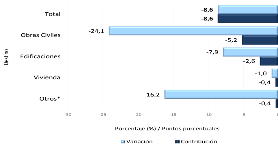
Gráfico 10. Variación y contribución año corrido del concreto premezclado, según destino Total nacional Enero – noviembre 2016 p / 2015
