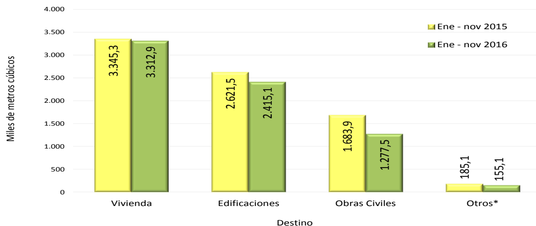
Gráfico 9. Producción concreto premezclado, según destino Total nacional Enero – noviembre 2016 p / 2015
