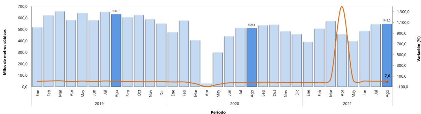
Gráfico 2. Producción de concreto premezclado (miles de metros cúbicos y variación anual) Total nacional Enero 2019 – agosto 2021 P
