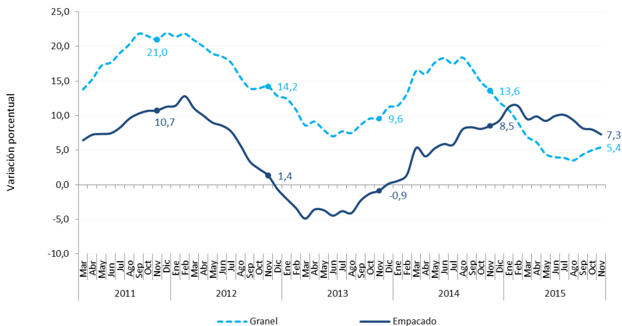
Gráfico 23 Variación acumulados móviles de doce meses de los despachos nacionales de cemento gris por tipo de empaque Total Nacional 2011 (marzo) – 2015 (noviembre) P
