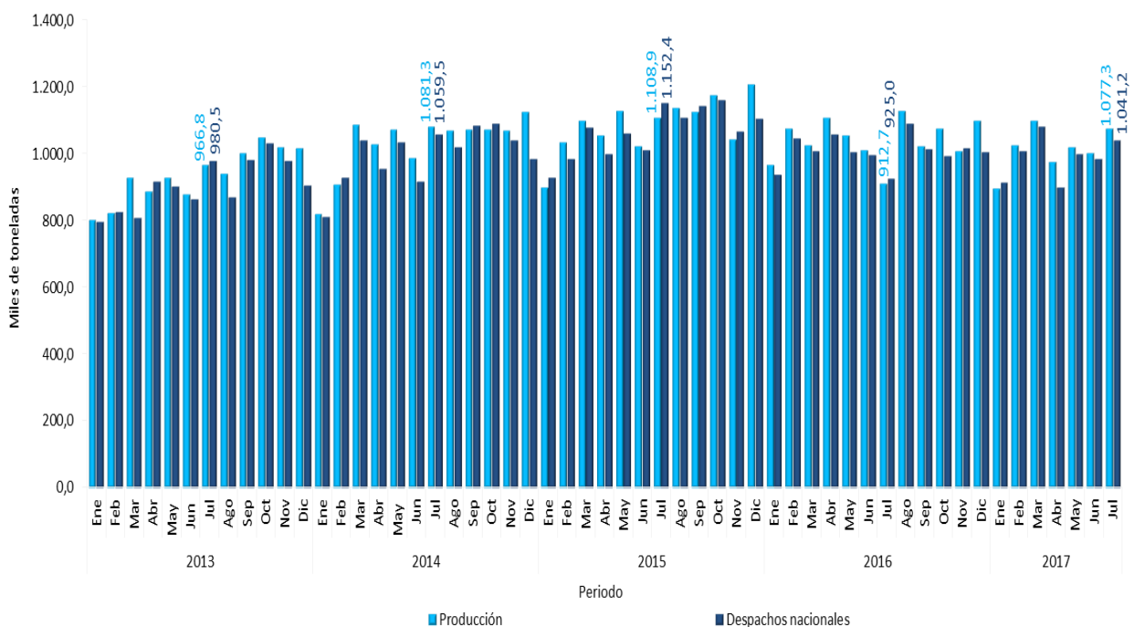
Gráfico 1. Producción y despachos mensuales de cemento gris Total nacional 2013 (enero) – 2017 (julio) p
