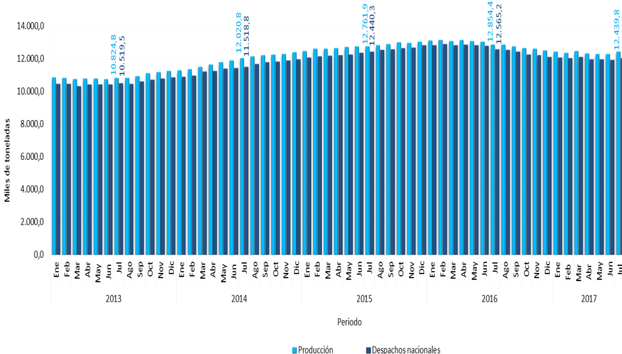
Gráfico 5. Producción y despachos nacionales de cemento gris acumulados doce meses Total nacional 2013 (enero) – 2017 (julio) p
