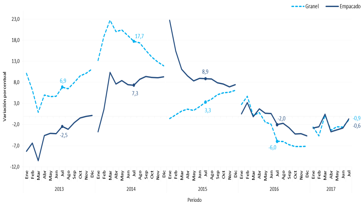
Gráfico 21. Variación año corrido de los despachos nacionales de cemento gris, según tipo de empaque Total Nacional 2013 (enero) - 2017 (julio) º
