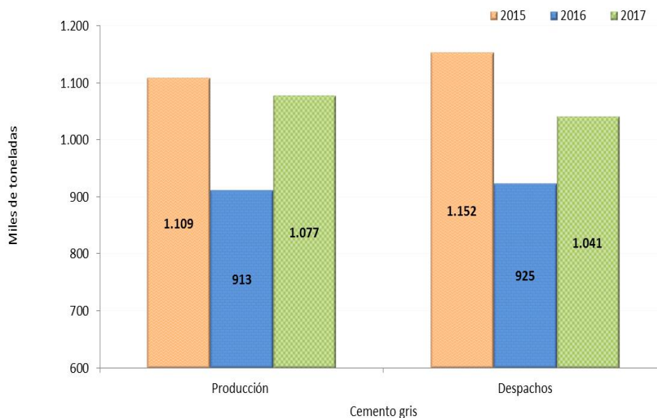
Producción y despachos de cemento gris Julio (2015-2017 P )
