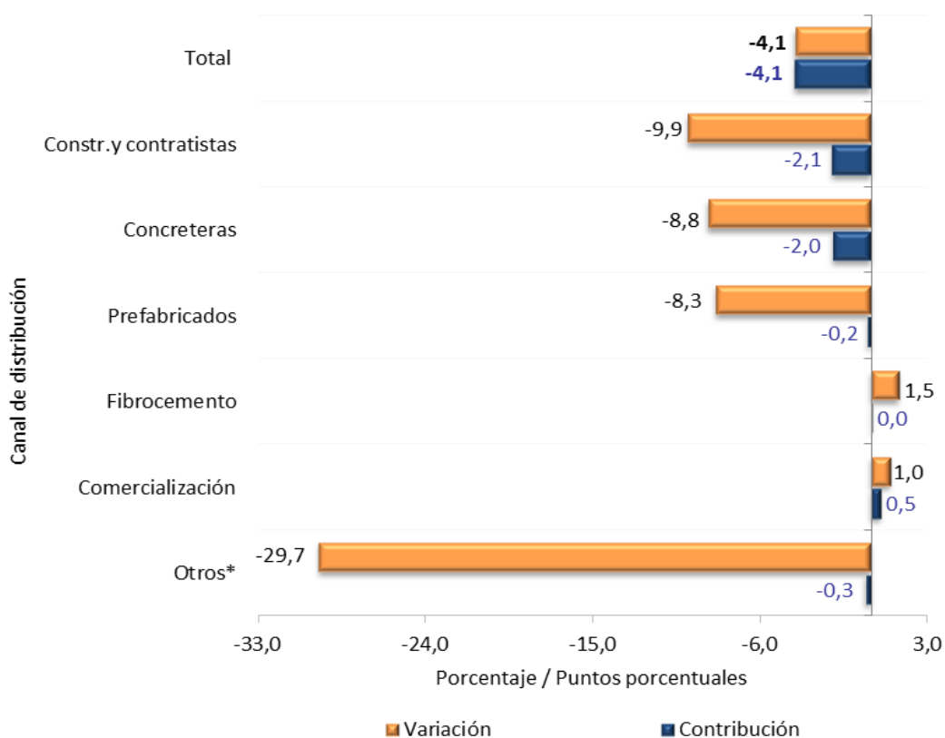
Gráfico 11. Variación y contribución acumulada doce meses de los despachos de cemento gris, según canal de distribución Total Nacional Agosto 2016 – julio 2017 p / agosto 2015 – julio 2016
