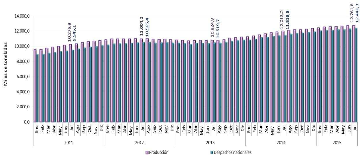
Gráfico 5 Producción y despachos nacionales de cemento gris Acumulados móviles de doce meses Total nacional 2011 (enero) – 2015 (julio) P
