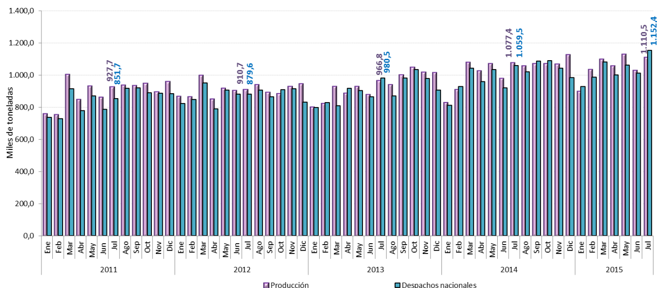
Gráfico 1 Producción y despachos mensuales de cemento gris Total nacional 2011 (enero) – 2015 (julio) P
