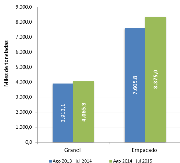
Gráfico 22 Despachos nacionales de cemento gris por tipo de empaque Total Nacional Agosto– julio (2014 – 2015) P
