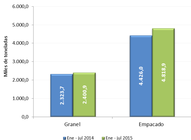
Gráfico 20 Despachos nacionales de cemento gris por tipo de empaque. Total Nacional Enero – julio (2014/2015) P
